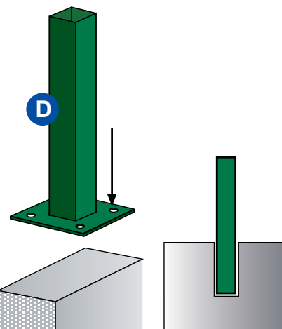
Sistemi di Fissaggio del montante.
