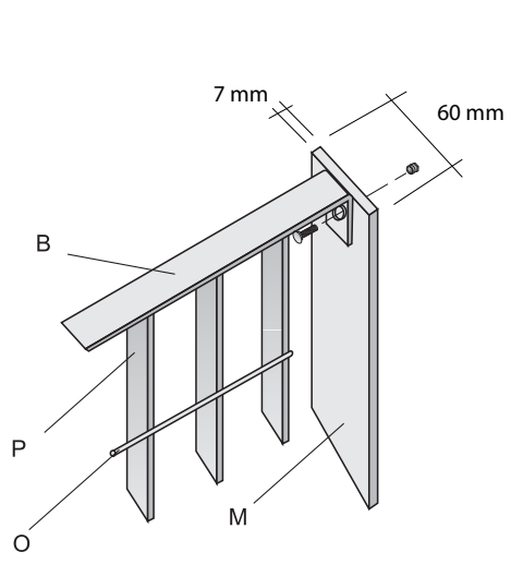
Montanti con doppia foratura per tratti in pendenza
